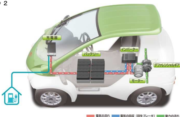
EVシステムイメージ
